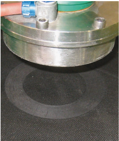
Illustration 8: Spécimen après l'essai d'abrasion
