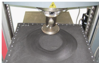
Illustration 2: Mesure de la déformabilité
