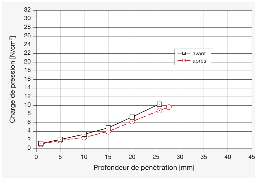
Illustration 4: Déformabilité en fonction de la pression d'appui
