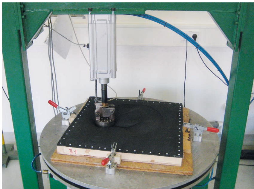
Illustration 5: La charge de la bande de roulement continue
